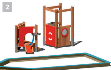
Spielschiff Dämpelnde Dorie 1780 & 0780 EM-D2-1780-* & EM-D-0780-* S. D-34
